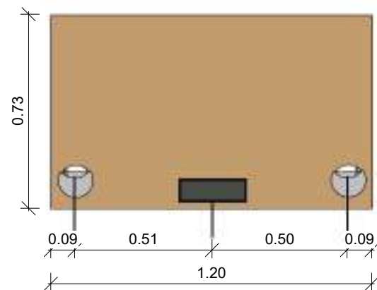
2 Planta Baixa 1 : 20
