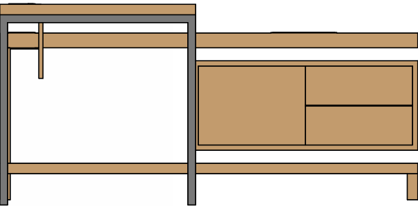
3 Vista Frontal 1 : 20
