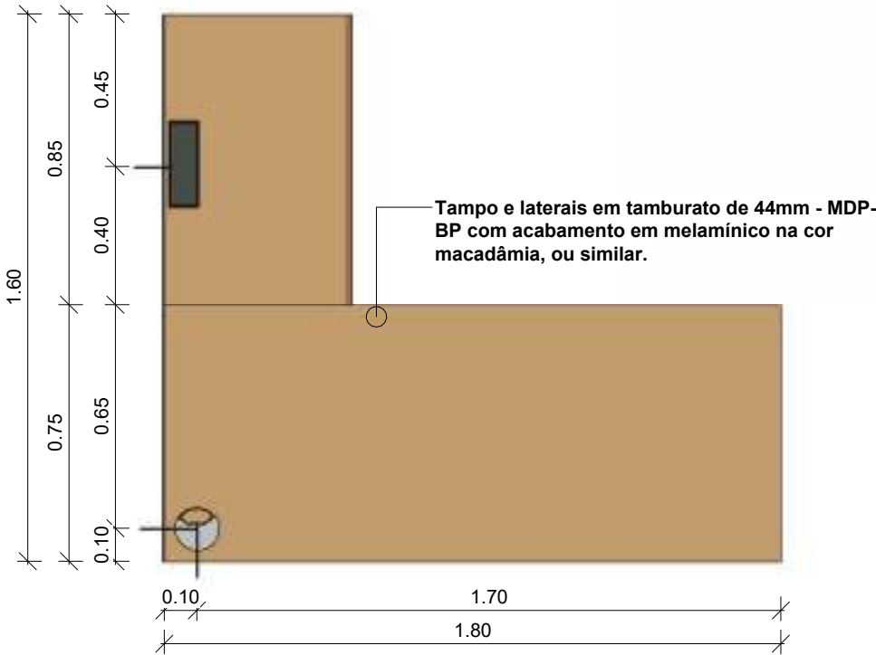
2 Planta baixa 1 : 20
