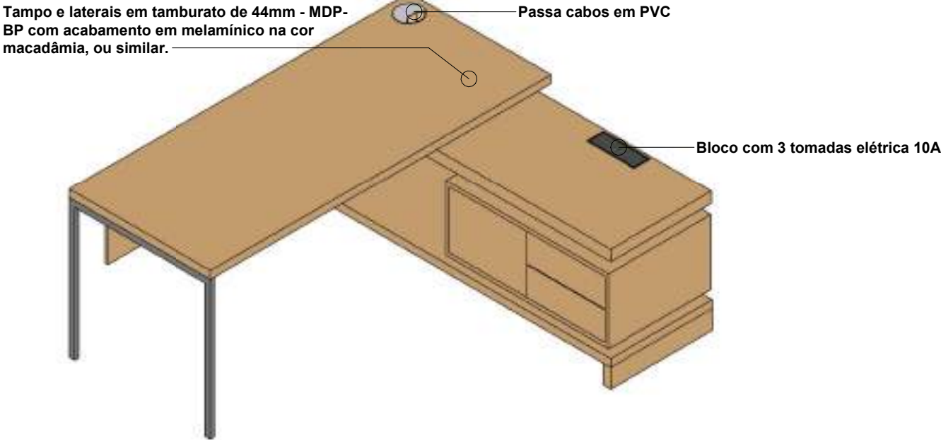
1 Perspectiva
